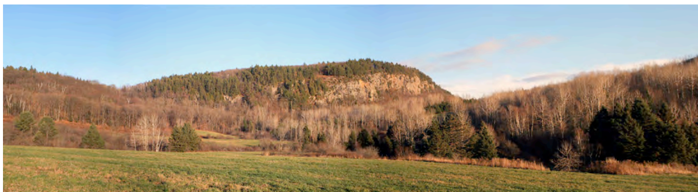
Falaise de la montagne Coupée à Saint-Jean-de-Matha, haute d'environ 1000 pi (304,80m). Panorama_1.jpg
